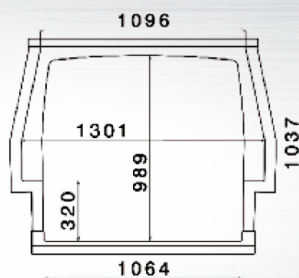
Vue arrière
