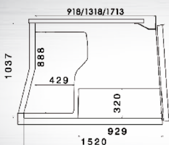
Vue côté
