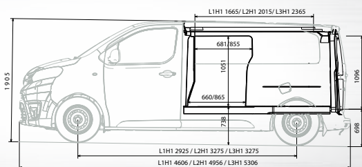
Vue côté
