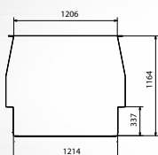
Vue arrière
